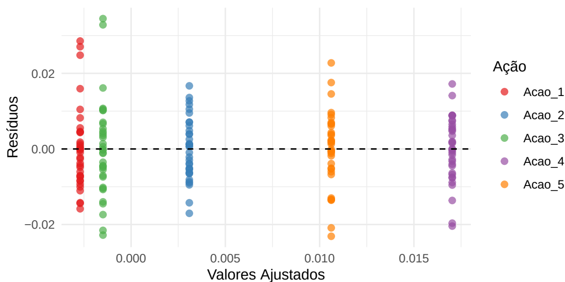
Figura 2: Resíduos pelos valores ajustados do modelo ANOVA
